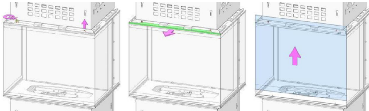
Obr. 3 Vyjmutí skla
