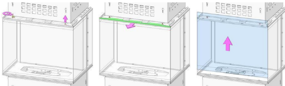
Рис. 3 Извлечение стекла
